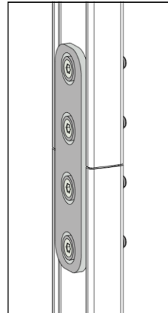
Sektion-Holmaußenverbinder
