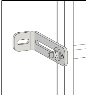
Befestigung der Leiter mit Gewindestange durch Sprosse
