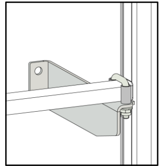
Befestigung der Leiter über Wandhalter mit Bügelschraube Sprosse
