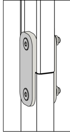
Leiteradapter 60 x 20 auf 60 x 25
