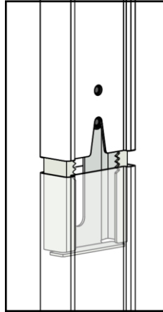
Versenkbarer Holminnenverbinder 60 x 20
