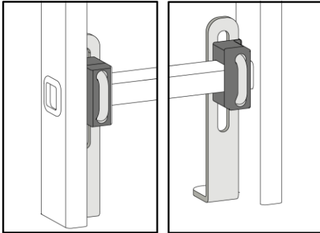
Bodenbefestigung an der Leitersprosse
