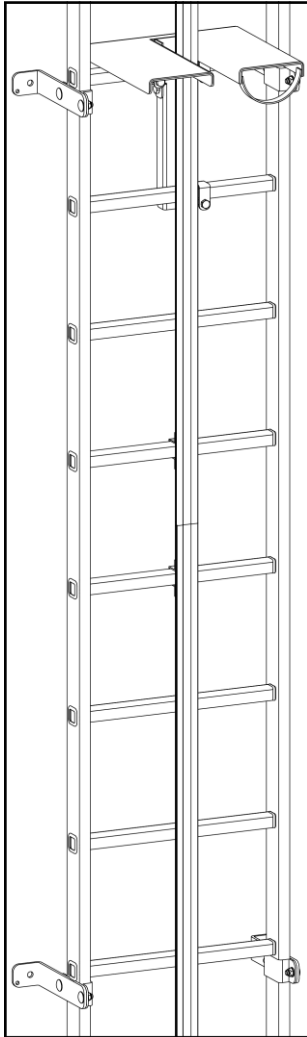
Aluminium-Steigleiter Holmprofil 72 x 25 mm
