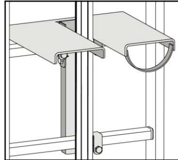
Ruhepodest geteilte Trittfläche (klappbar)
