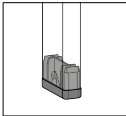
Endkappe im Leiterholm
