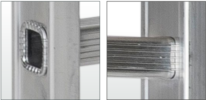
Links: Doppelt verwulstete Holm-Sprossenverbindung Left: Double beaded rail-rung connections
